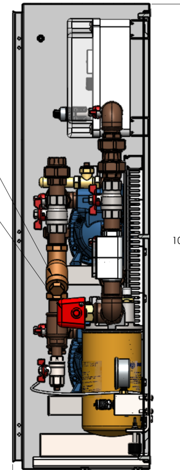
SECTION A-A
